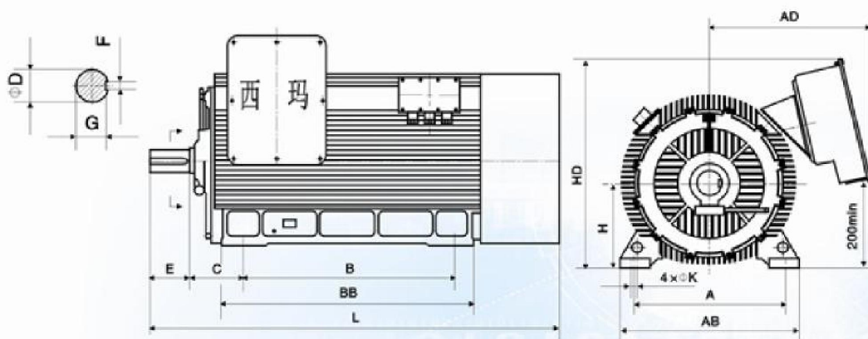
Y2系列10KV三相异步电动机 (机座号450~560) 外形安装尺寸图
